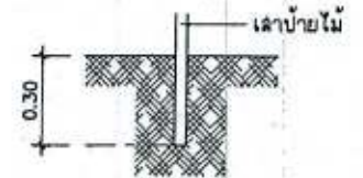
ขยายการติดตั้งเสา ปสล.ชั่วคราว SCALE 1:20
