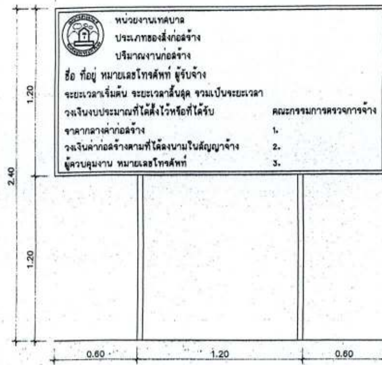
แบบป้ายประชาสัมพันธ์ชั่วคราว SCALE 1:20
