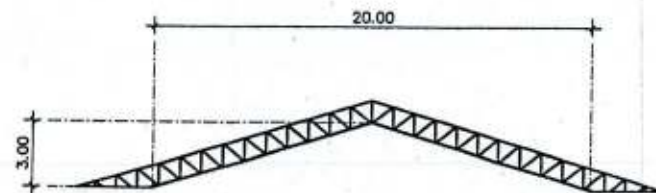
แปลนโครงร่างใหม่ SCALE 1:100
