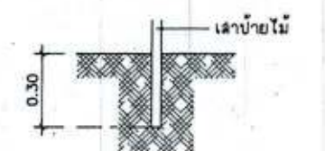
ขยายการติดตั้งเสา ปชฉ.ชั่วคราว SCALE 1:20
