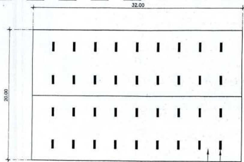
แปลนโครงร่างเดิม SCALE 1:100
