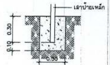
ขยายการติดตั้งเสา ปสล. SCALE 1:20
