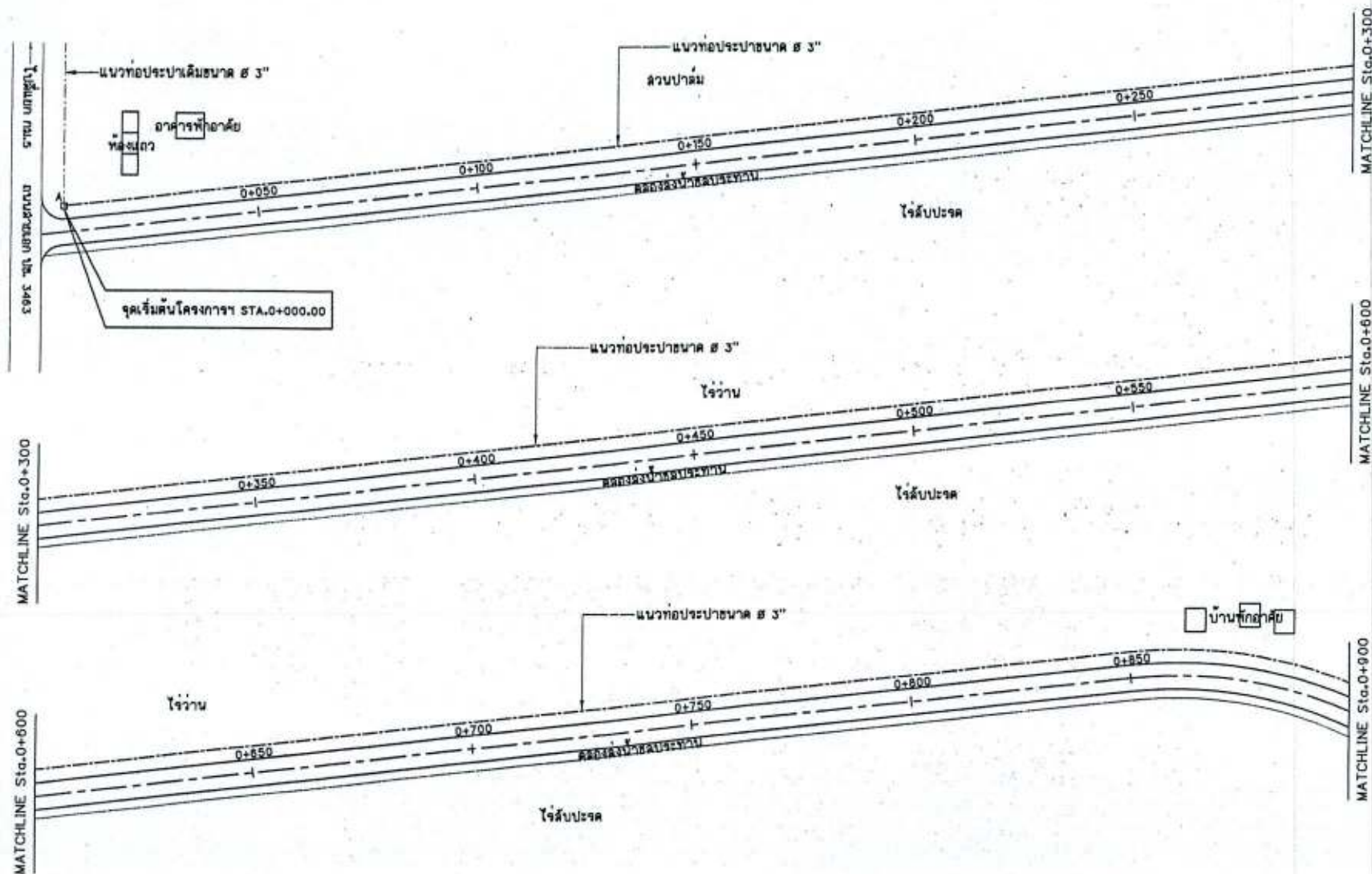
แปลนแนววางท่อประปา SCALE 1:1000
