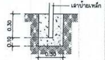
ขยายการติดตั้งเล้า ปชส. SCALE 1/20
