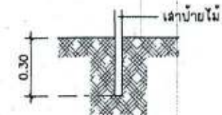
ขยายการติดตั้งเสา ปชส.ชั่วคราว SCALE 1:20
