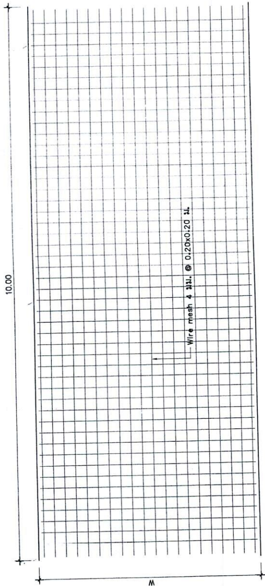
แปลนแสดงการเสริมเหล็กลานคอนกรีต SCALE 1:50
