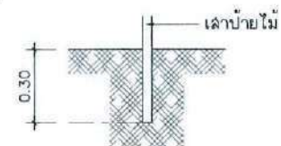
ขยายการติดตั้งเสา ปชส. SCALE 1:20
