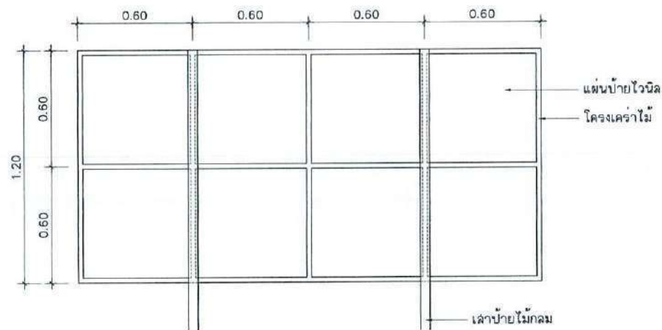
แบบแสดงโครงเคร่าไม้ป้ายประชาสัมพันธ์ SCALE 1:20
