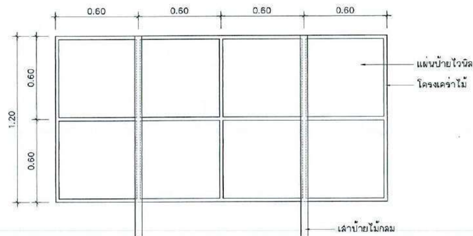
แบบแสดงโครงคร่าวไม้ป้ายประชาสัมพันธ์ SCALE 1:20
