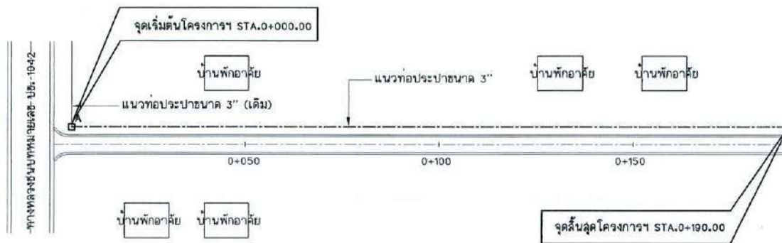
แปลนแนววางท่อประปา SCALE 1:1000
