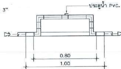
ประตูน้ำ SCALE 1:20
