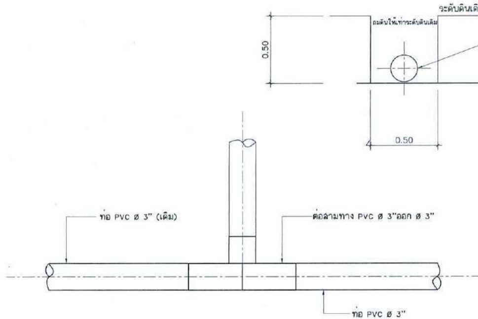
แบบการต่อลำทาง PVC SCALE 1:20
