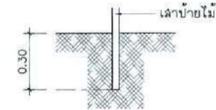
ขยายการติดตั้งเสา ปชส. SCALE 1:20
