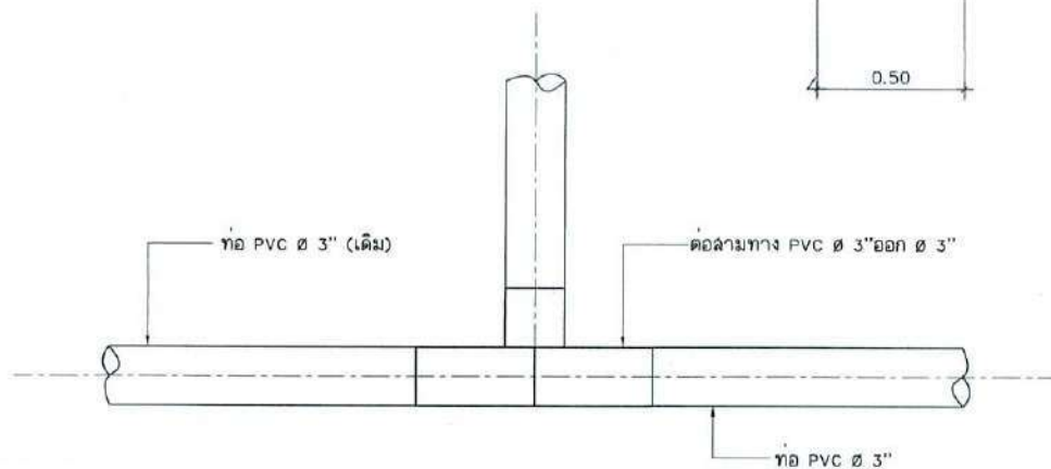
แบบการต่อลำทาง PVC SCALE 1:20
