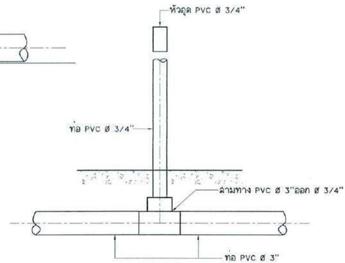
แบบการต่อลำทางลด SCALE 1:20
