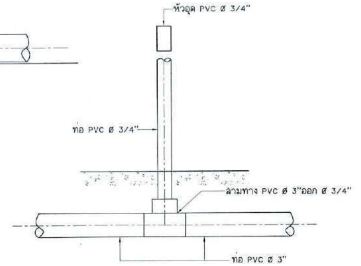
แบบการต่อลำทางลด SCALE 1:20
