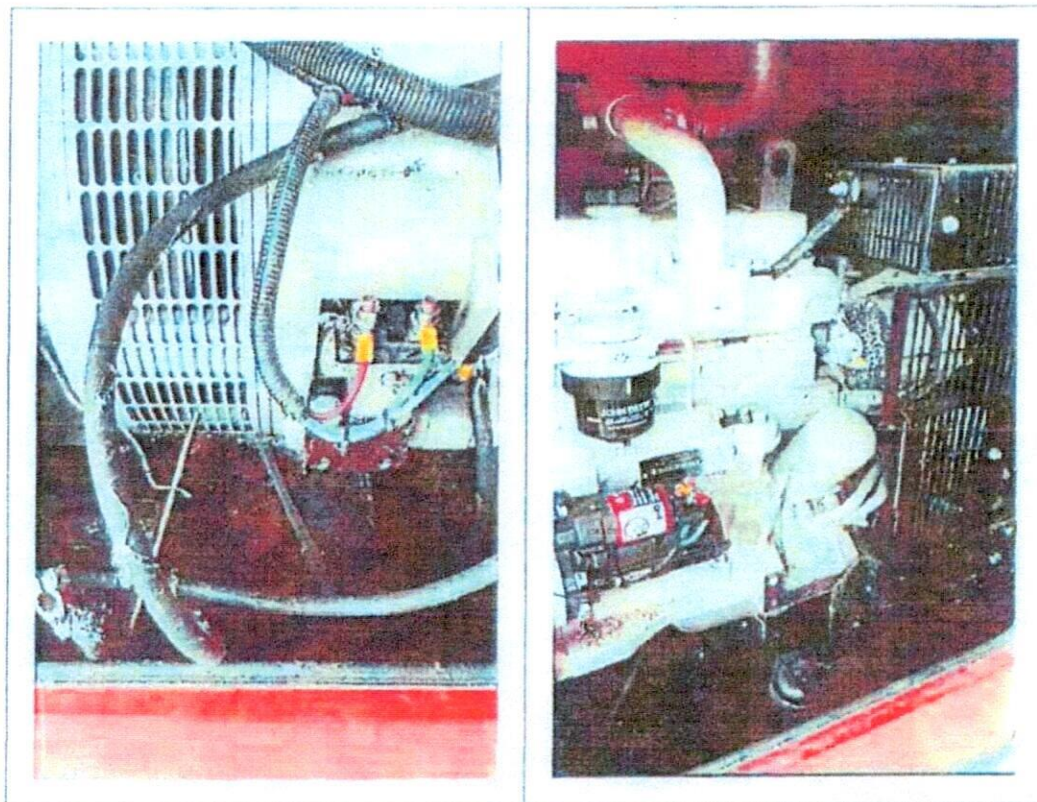
ภาพถ่ายบริเวณ Underpass กม.298+826 ความเสียหายแบตเตอรี่สาร์ทเครื่องสูบน้ำสูญหาย
